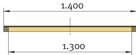
Rückwand (Draufsicht)
