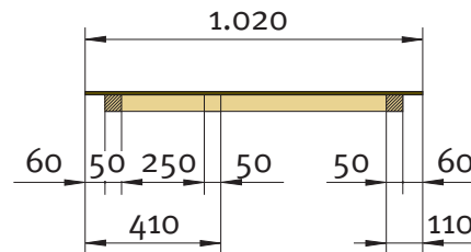
Seitenteil (Draufsicht)
