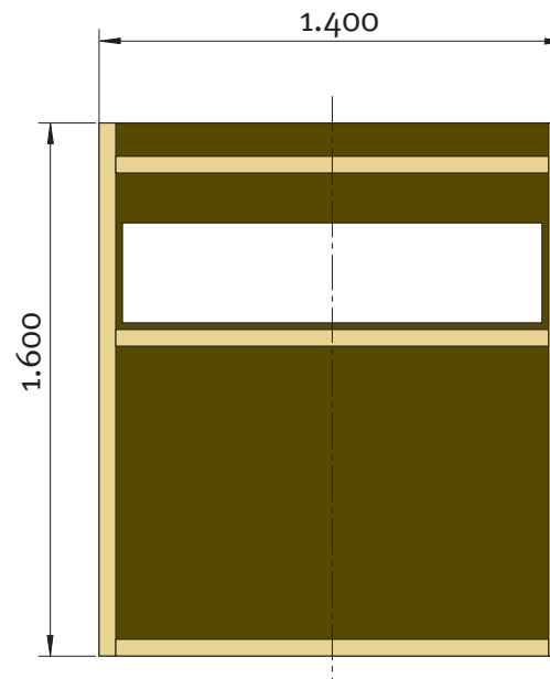
Frontwand (innen)
