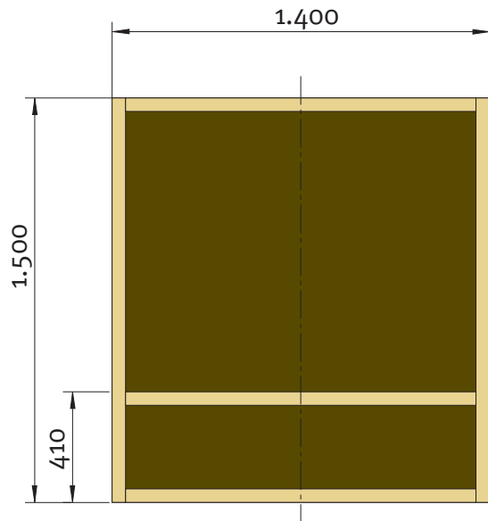
Rückwand (innen)
