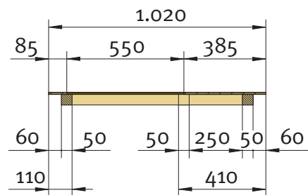
Seitenteil (Draufsicht)
